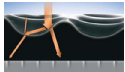
Geringe Reflexion an der Luft-Glas-Grenzfläche
